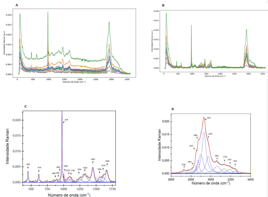
FIGURA 1. PROCESSAMENTO DOS DADOS. A - ESPECTROS ORIGINAIS, B - ESPECTROS ORIGINAIS MAIS A LINHA DE BASE. C E D - ESPECTROS DAS AMOSTRAS. AS SETAS INDICAM OS PICOS RAMAN IDENTIFICADOS.
