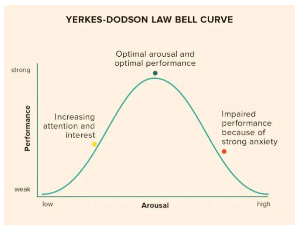
Figura 1 - Lei de Yerkes-Dodson: Relação entre Ansiedade e Desempenho
