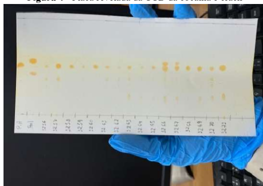
Figura 4 - Placa revelada da CCD da cocaína e crack
